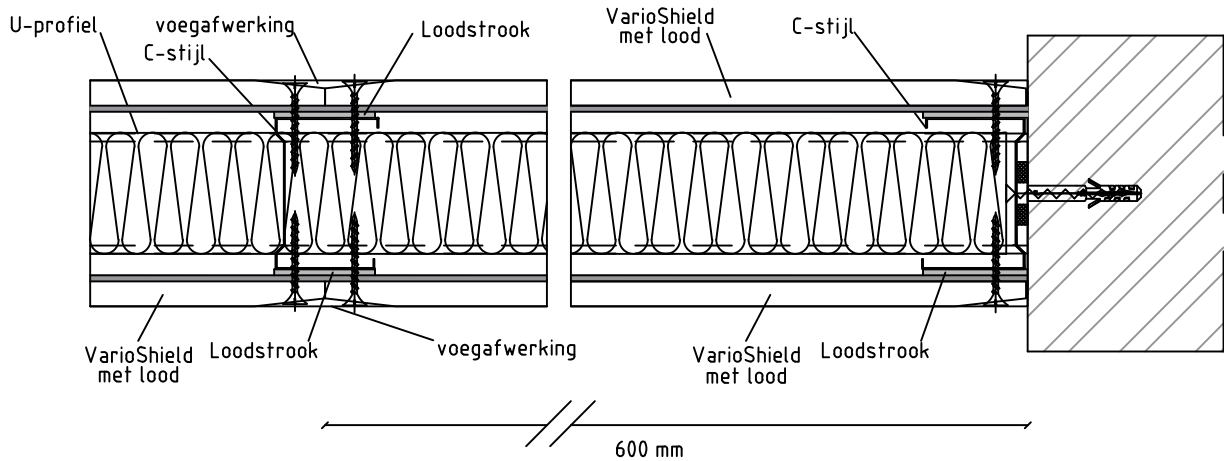
Dwarsdoorsnede
