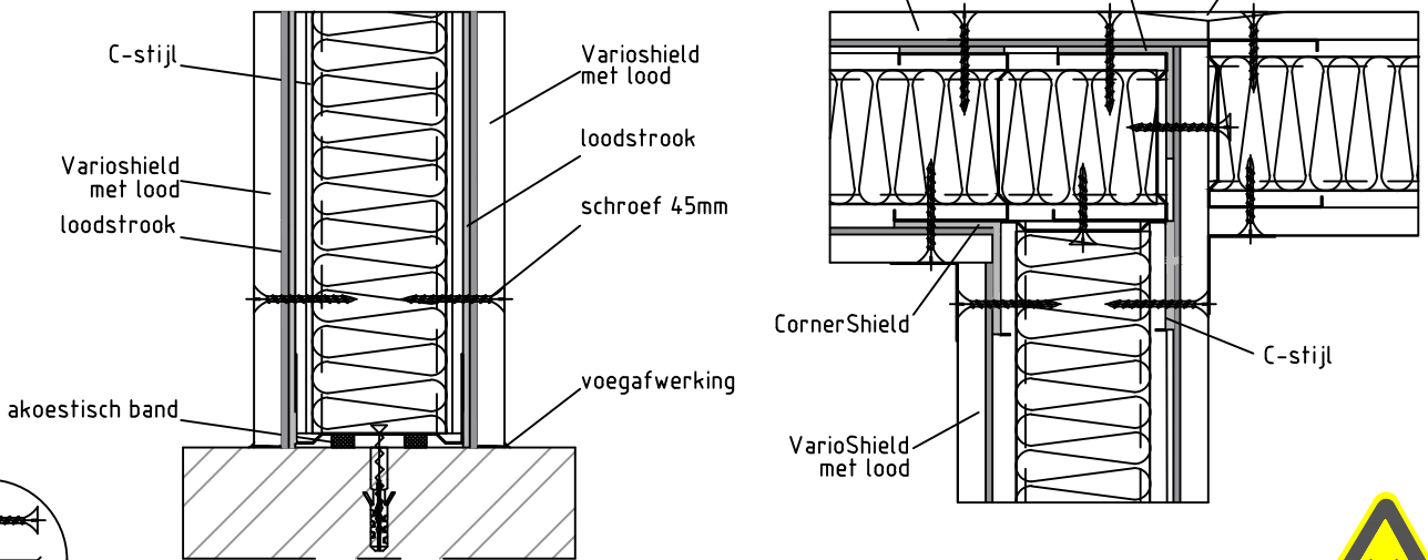
Onderaansluiting
