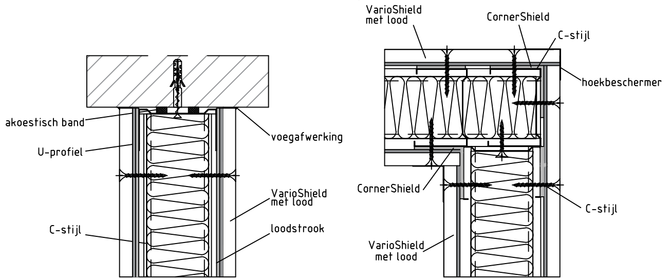
Bovenaansluiting
